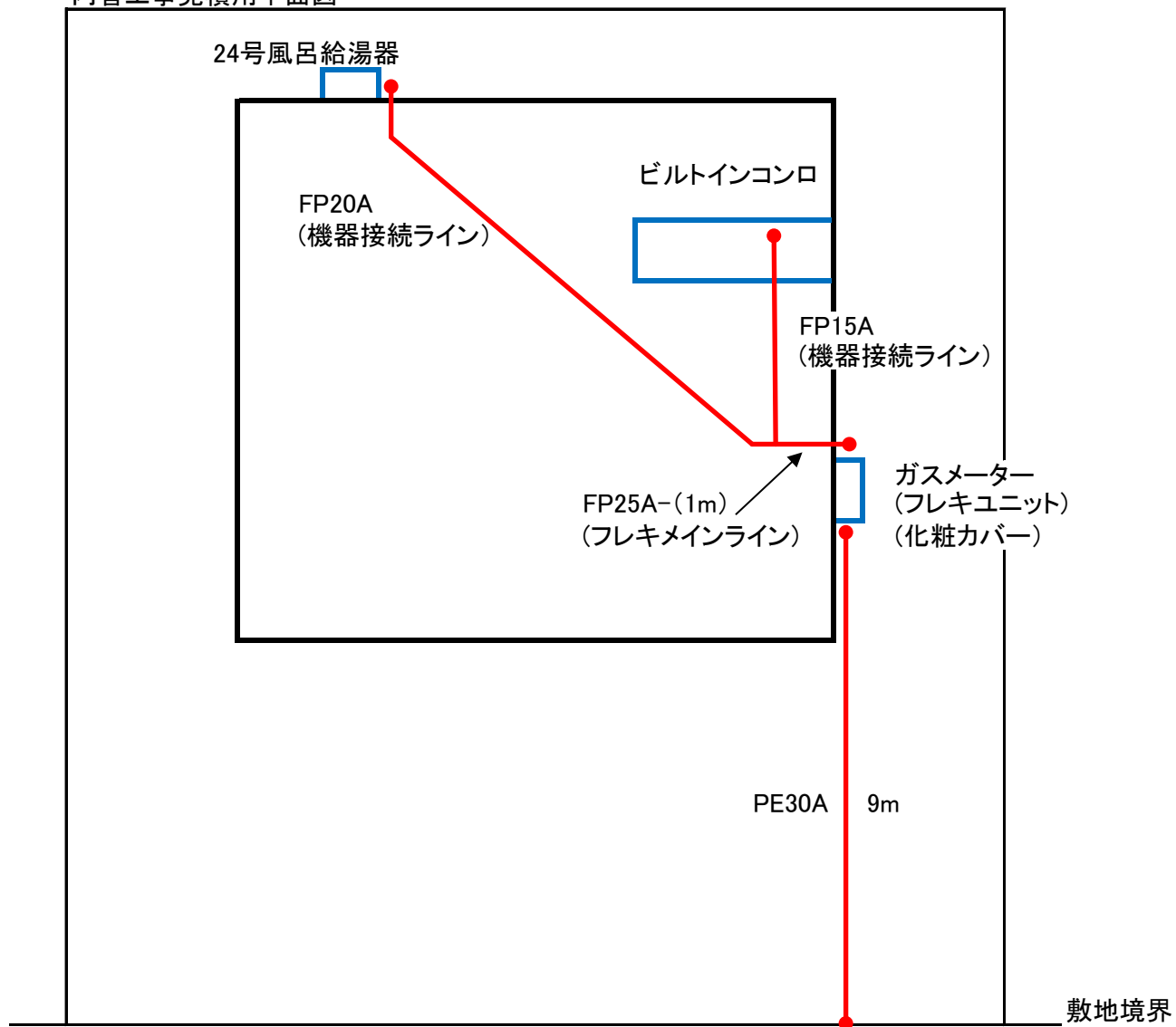
内管工事見積用平面図
