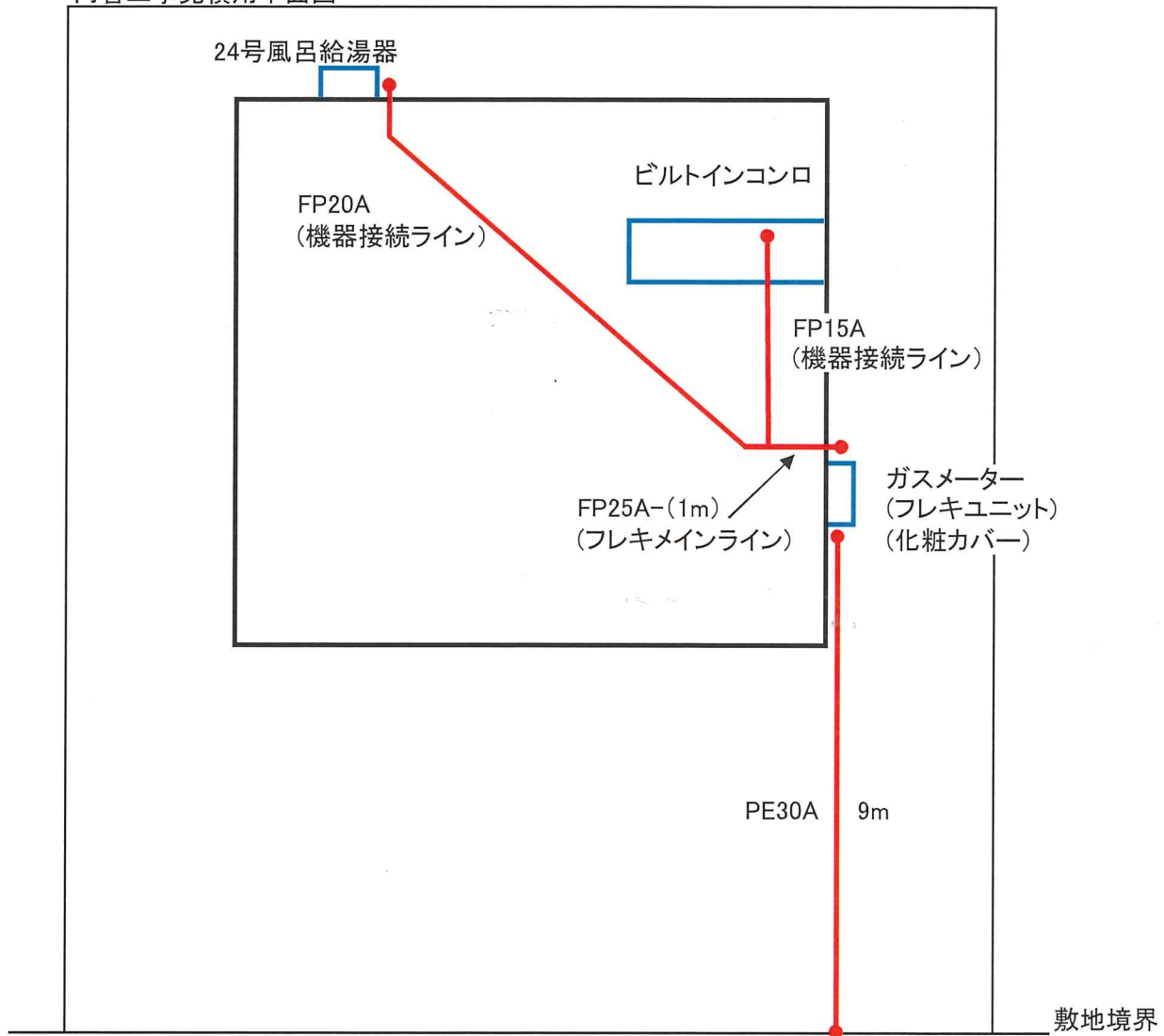
内管工事見積用平面図
